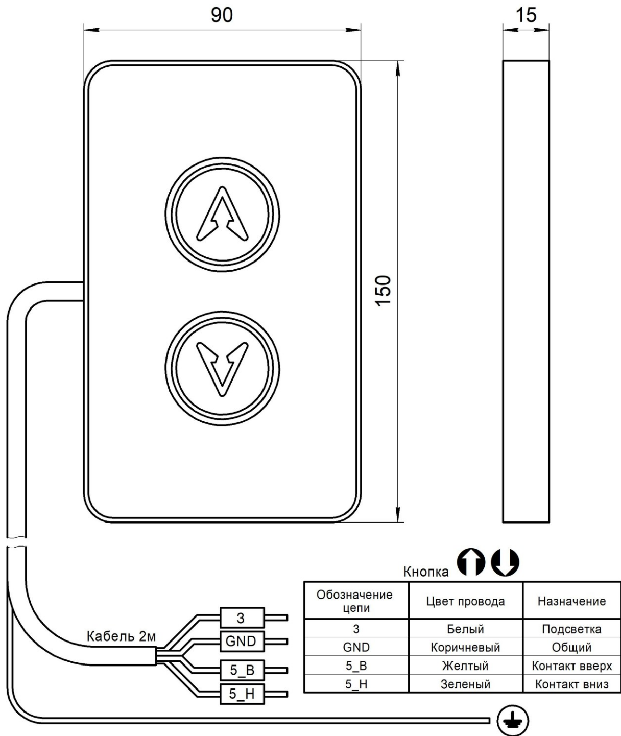
Рис.1 Внешний вид, габаритные и установочные размеры Вызывного поста ОНИКС НШЕК.468381.125
